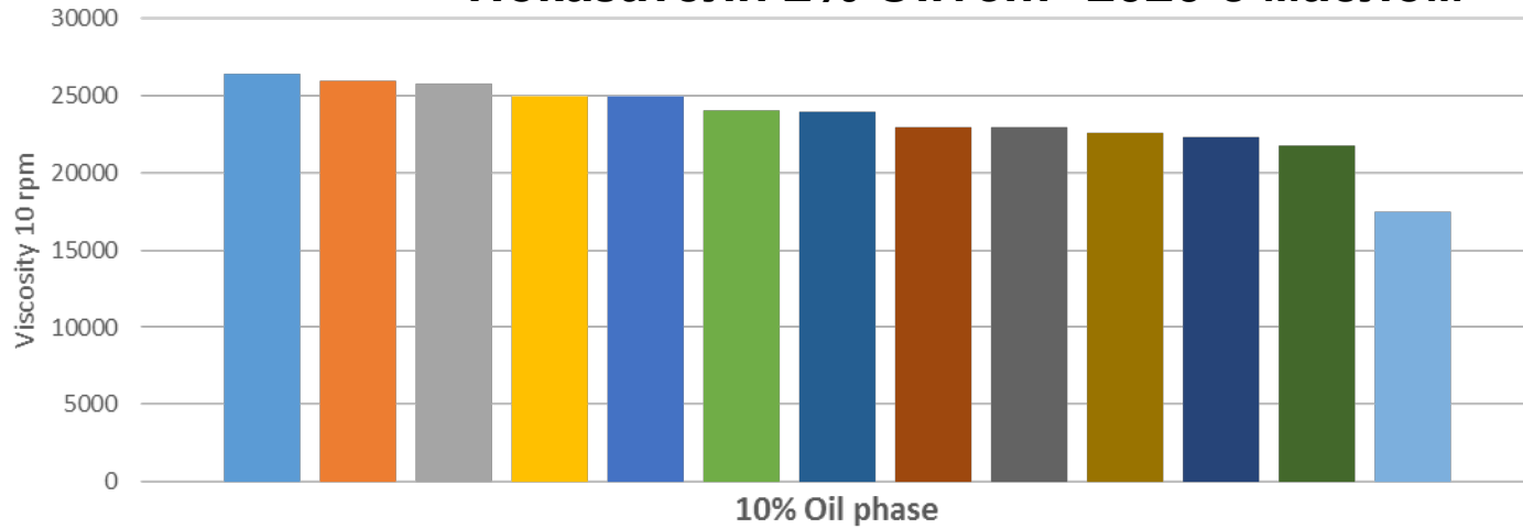
Показатели 2% Olivem ® 2020 с маслом
